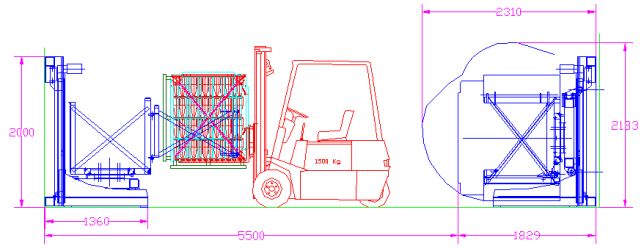
Côtes du remueur. Côtes au déchargement. Côtes maxi. au remuage.
